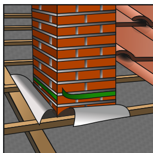
Wiatroszczelne połączenie podkładu z kominem za pomocą wodoodpornej taśmy klejącej z kauczuku butylowego Gerband 970
