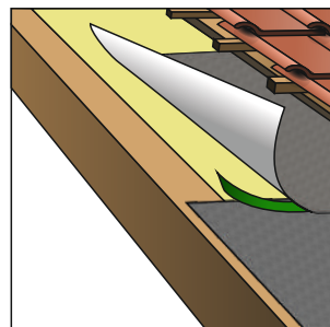
Wiatroszczelne klejenie w obszarze zakładów membran krytych poliakrylową taśmą klejącą Gerband 970
